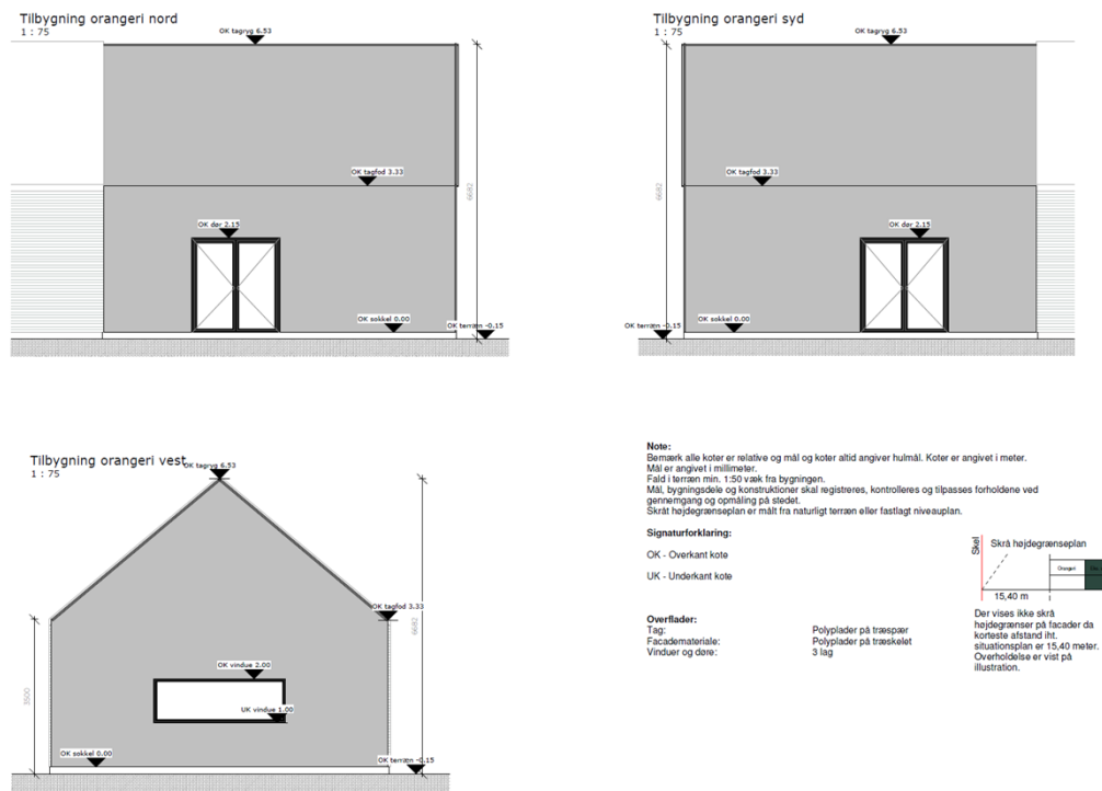
Facader af drivhuset set fra nord, syd og vest
