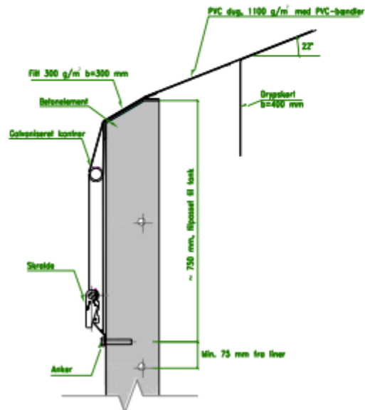
DETALJE A
