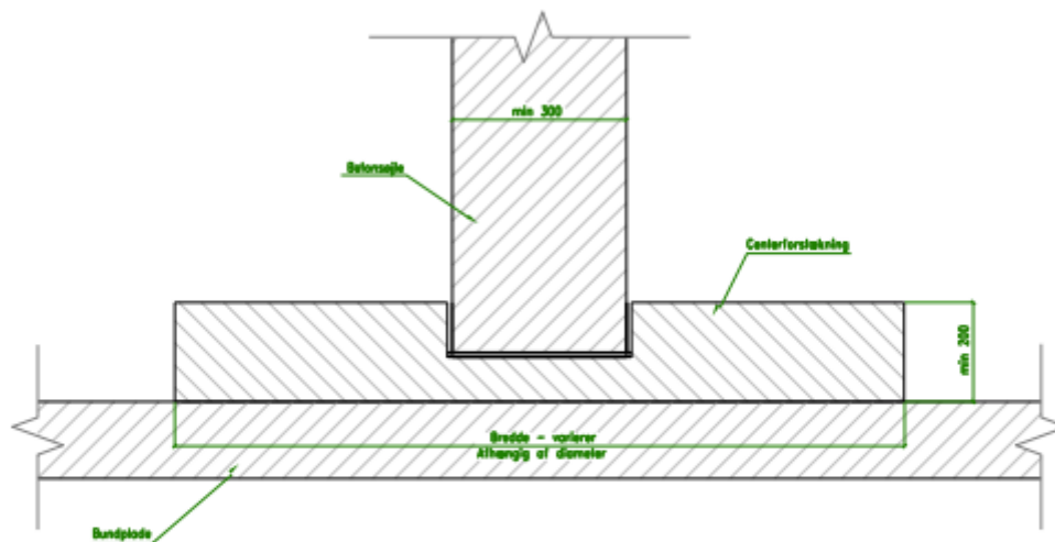
DETALJE B
