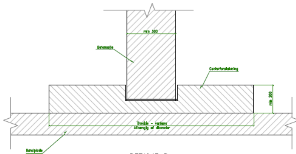
DETALJE B
