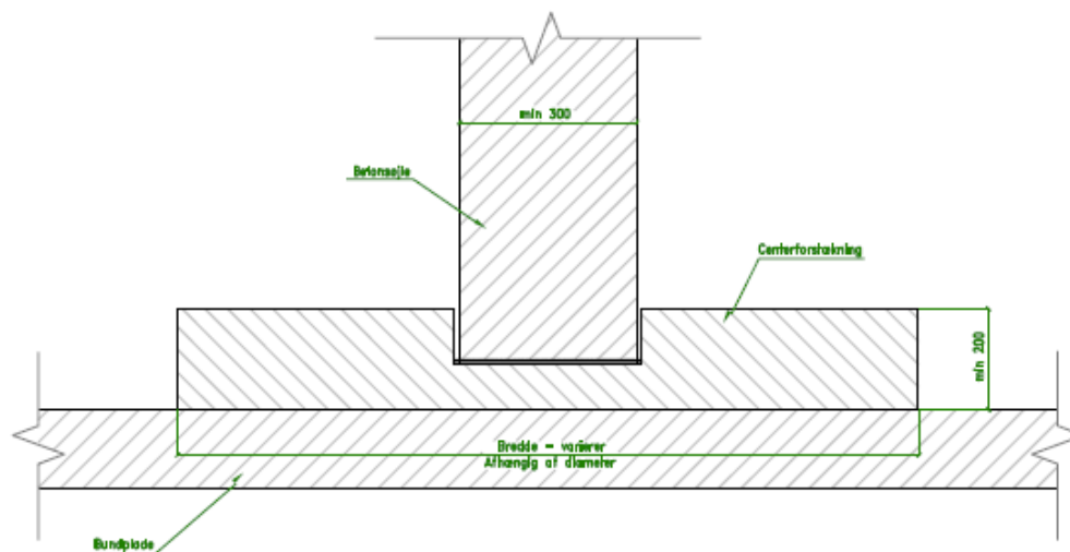
DETALJE B
