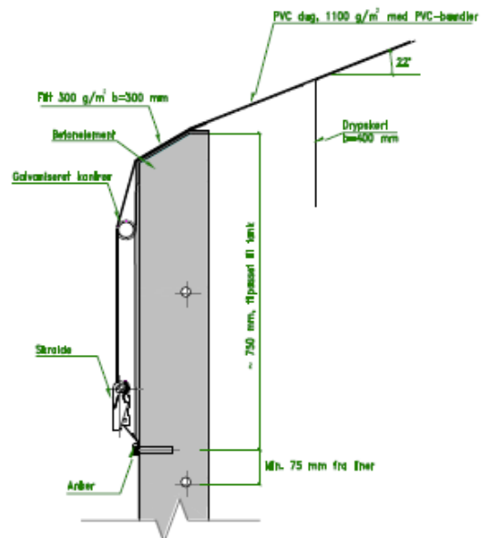
DETALJE A
