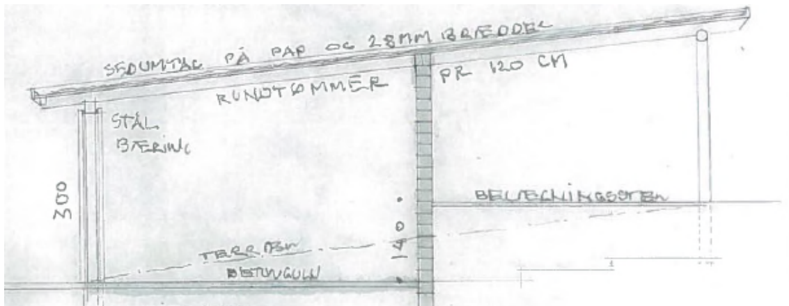
Figur 2: Snit der viser bygningens placering i terræn
